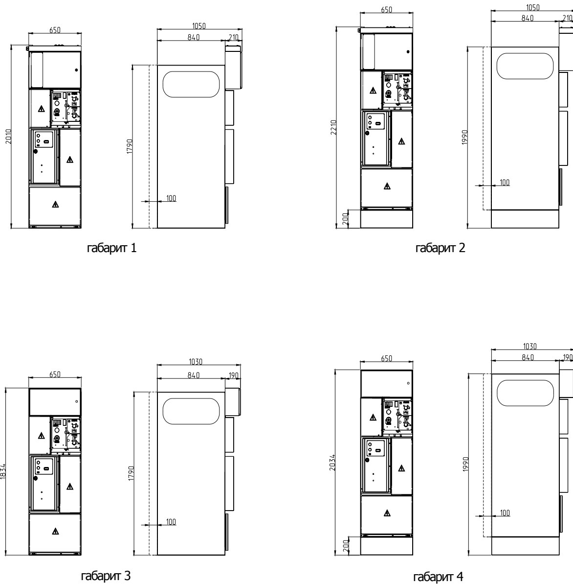
Рис. 2. Габаритные размеры КСО с шириной корпуса 650 мм (схемы №№ 10.2, 10.3)
